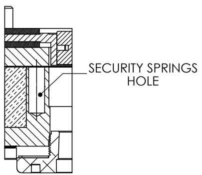
SEZIONE B-B SCALA 1 : 2
