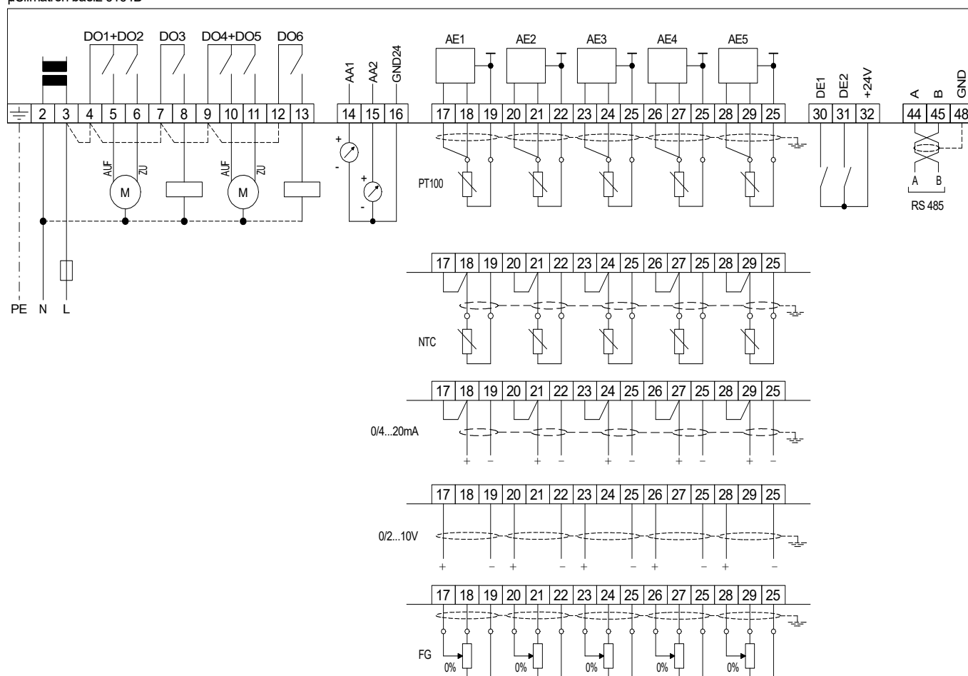
Beispiel-Anschlussplan: 6164B, Schalttafel-Gerät
