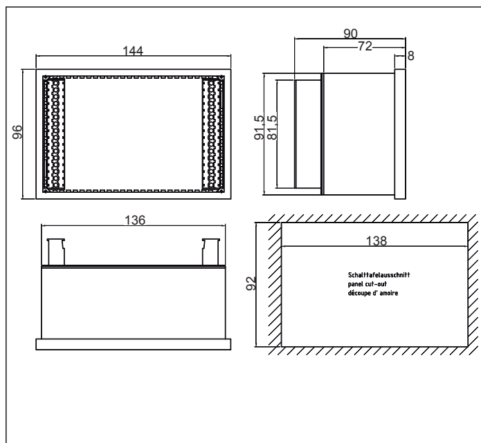
Abmessungen 6164B, Schalttafel-Gerät
