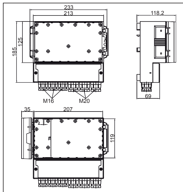
Abmessungen 6164B-W2, Wandaufbau-Gerät
